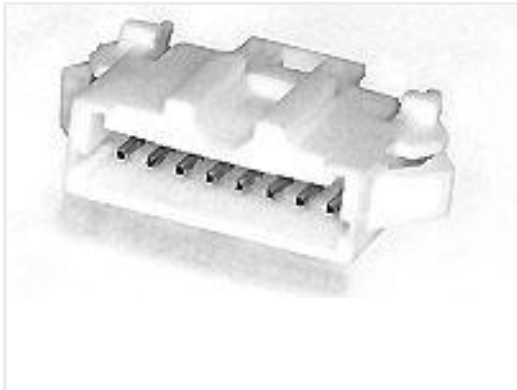
TE 产品编号292215-5 MINI CT SGL RELAY 5P NAT
