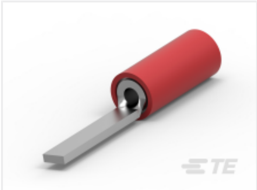
TE 产品编号150730 22-16 PIDG TAB 3,3/3
