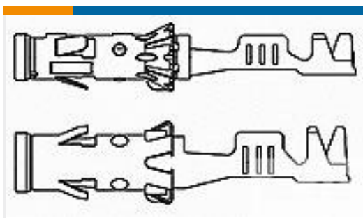
TE 产品编号929974-8 2,5MM ST-KONT EDS
