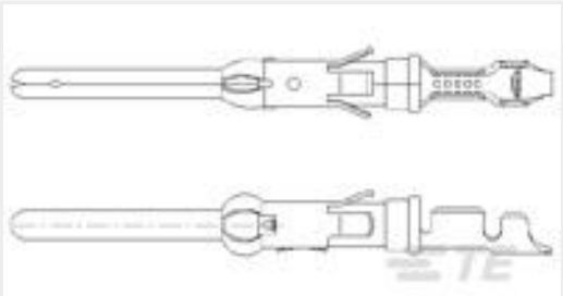
TE 产品编号163085-2 .062 DIA PIN ASS 3+
