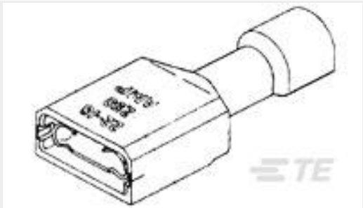
TE 产品编号3-520412-2 ULTRA-FAST 187 ASY REC 16-14 AWG TPBR
