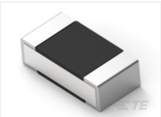
TE 产品编号5-2176307-4 RP 1E 0.1W 44K2 0.1% 25PPM 5K RL
