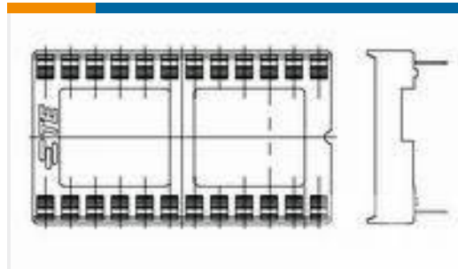
TE 产品编号1-2199299-5 40P,DIP SKT,600 CL,LDR,PB FREE
