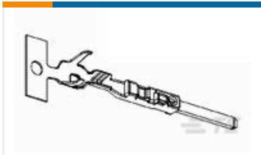
TE 产品编号2141116-3 MCON 1.2 CB TAB SWS AG
