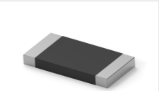
TE 产品编号9-2176422-1 TLRP 2512 3.0W R060 1% 75PPM 4K RL
