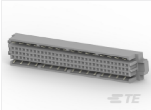
TE 产品编号 536154-5 096 ENHNCD EURO RECPT ST ASSY
