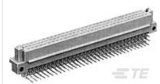
TE 产品编号 5536407-5 ASSY,PIN,EUROCARD,TYPE C/2,LEAD-FREE,48
