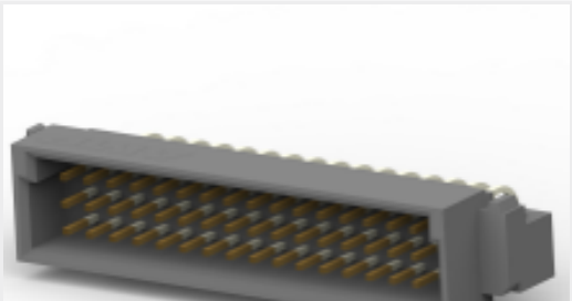
TE 产品编号 5148474-1 ASSY,PIN,EUROCARD,TYPE R/2,LEAD-FREE,48
