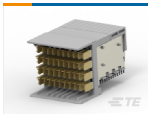
TE 产品编号 6469183-1 HMZD 3PR RA HDR 60P ASSY LF
