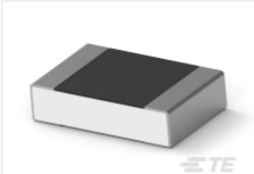
TE 产品编号3-2176381-0 RQ 0805 24K9 0.1% 10PPM 5K RL
