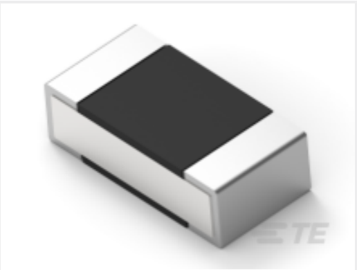
TE 产品编号2176308-1 RP 1E 0.1W 133K 0.1% 25PPM 5K RL
