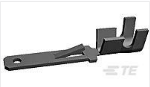
TE 产品编号42460-2 FF 250 TAB 18-14AWG TPBR
