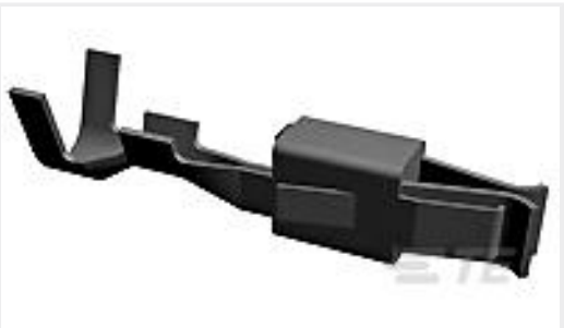
TE 产品编号2-929939-1 JPT REC 2.8 Contact SWS Au
