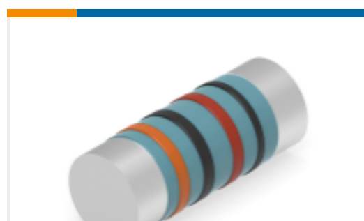
TE 产品编号4-1879283-0 MELF SMA 56K 1% 50PPM 1W 0207
