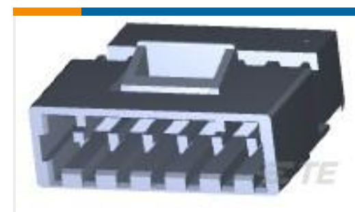
TE 产品编号3-641439-6 06P MTA156 PST CON ASSY LF
