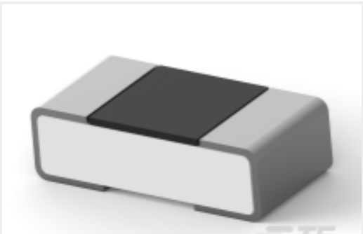
TE 产品编号6-2176363-3 RQ 0402 1K91 0.1% 10PPM 5K RL
