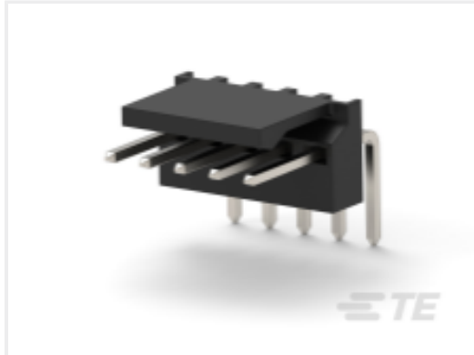
TE 产品编号 CAT-104MTA-NRTHH PCB Header: Nylon, Right Angle, 2.54 mm
