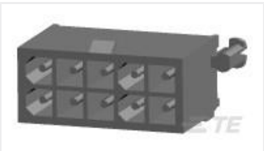
TE 产品编号1-770743-1 10P MINI UMNL HDR ASSY VRT LF
