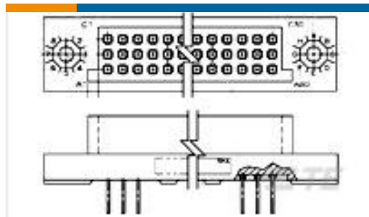
TE 产品编号448006-1 3 ROW BOX RECP 120 POS
