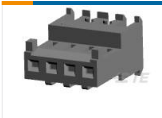
TE 产品编号3-644563-4 04P MTA100 CONN ASSY F/T 24AWG
