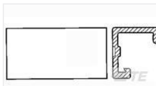
TE 产品编号174200-1 250 FASTON HSG.,REC.,3 POS, NATRUAL
