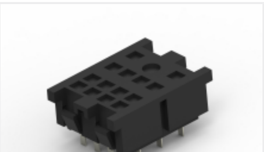
TE 产品编号1419106-3 27E023=SOCKET,KH,14,PCB,PHEN,BL
