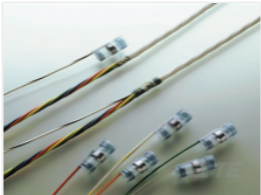
TE 产品编号223853N001 S02-17-R-95CS928
