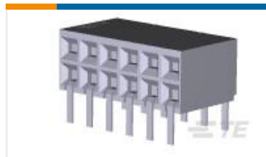
TE 产品编号5535512-1 12 MODII HORZ DR CE
