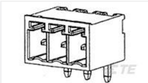
TE 产品编号284513-8 8 POS TERMI-BLOK HDR 900 POL.
