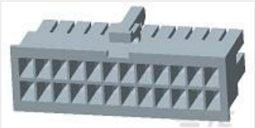
TE 产品编号1-1969614-0 10P RCPT VAL-U-LOK V0
