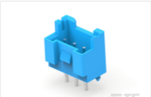
TE 产品编号2-2338245-3 EP2.5 HDR 3P VERT BOSS,BLUE,UL
