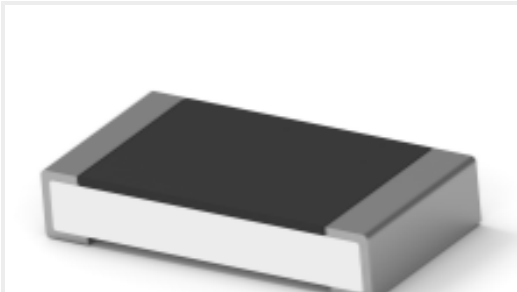
TE 产品编号9-2176391-2 RQ 1206 110K 0.1% 10PPM 5K RL
