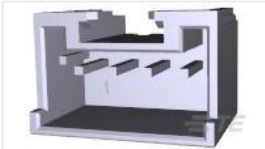
TE 产品编号917782-1 2.5 S.D.L POST HDR ASY 4P STD
