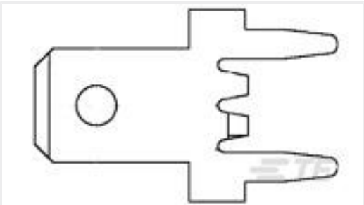
TE 产品编号63982-1 187 FASTON TAB TPBR
