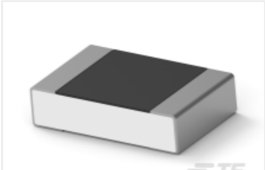
TE 产品编号2-2176376-4 RQ 0805 21K5 0.1% 10PPM 1K RL
