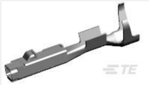
TE 产品编号1670146-2 MCON 1.2 CB REC SWS AU
