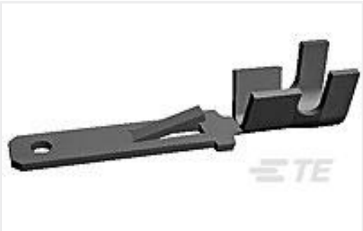
TE 产品编号170041-1 FF 110 TAB 20-16AWG BR LP
