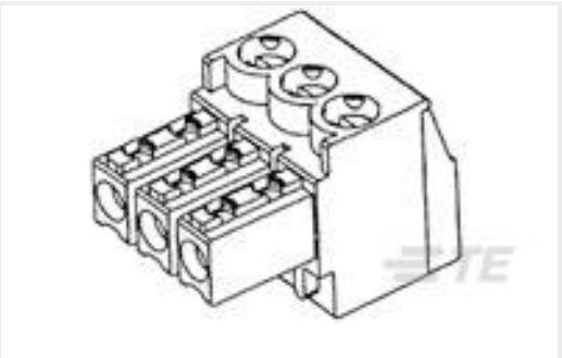
TE 产品编号1-284506-0 10 POS TERMI-BLOK PLUG STAC 3,
