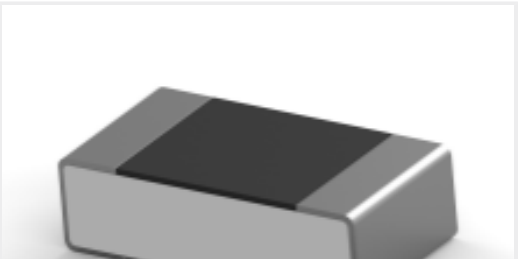
TE 产品编号2176370-8 RQ 0603 511R 0.1% 10PPM 5K RL
