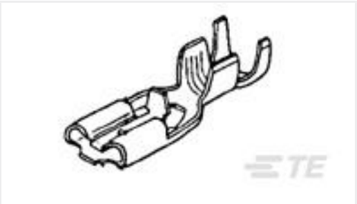
TE 产品编号170330-1 PL MKII 187 REC 24-20AWG PTBR LP
