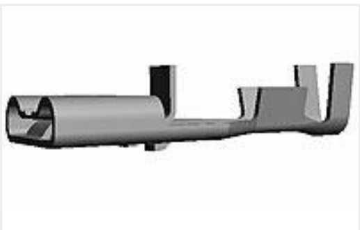
TE 产品编号170328-1 250 PL MKII REC. 18-14AWG PTBR
