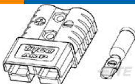
TE 产品编号1445999-2 AMP Power 120A Con KIT,4 AWG, BLUE
