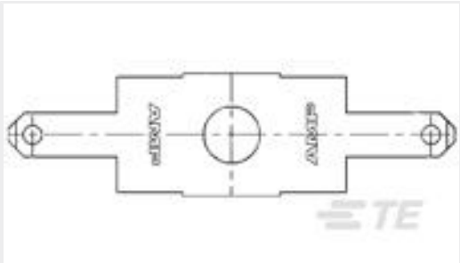
TE 产品编号62628-1 100 FASTON TAB TPST
