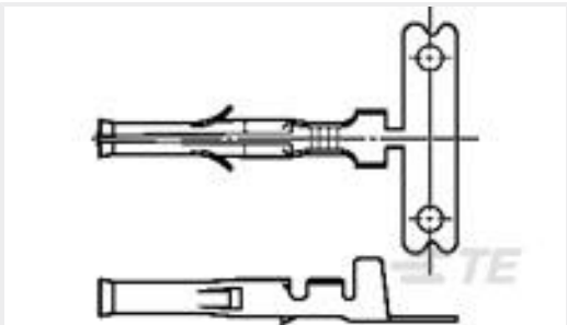
TE 产品编号350628-1 .062 COMM P&S SOK 18-24 PTPBR
