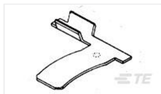
TE 产品编号62214-2 BRSH CONT AMPLIVAR 22-17 PHBZ
