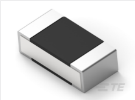
TE 产品编号2176309-5 RP 1E 0.1W 11R 0.1% 25PPM 1K RL
