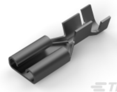
TE 产品编号 62137-2 187 FASTON REC 20-16 TPBR
