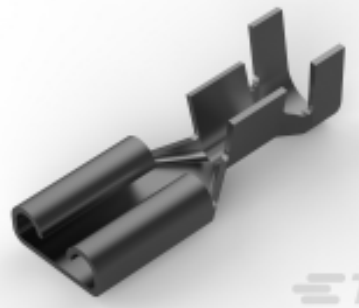
TE 产品编号 42452-2 187 FASTON REC 20-16 AWG TPBR
