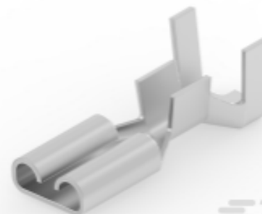
TE 产品编号 60487-2 187 FASTON REC 18-16 AWG TPBR
