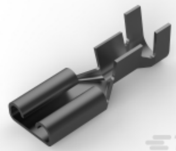
TE 产品编号 42452-5 187 FASTON REC 20-16 AWG TPBZ
