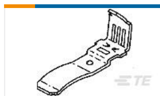
TE 产品编号62009-1 BRUSH CONTACT TAB 20-14 AWG PHBZ
