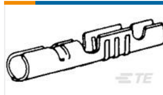
TE 产品编号42101-2 PIN RECEPTACLE 18-16 AWG TPBR
