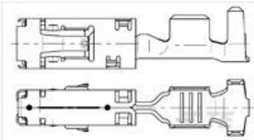
TE 产品编号967543-1 SENSOR FLA-KONT 2,8
