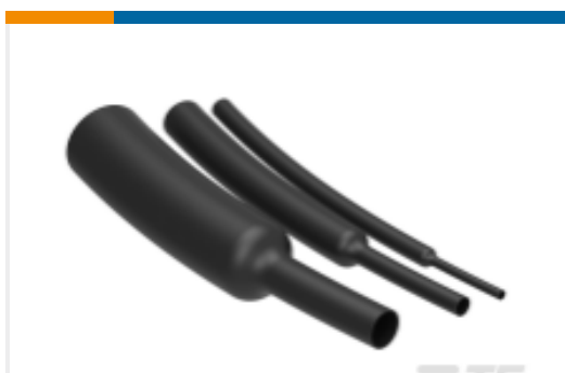
TE 产品编号5069864018 CGPT 2:1 热缩管
