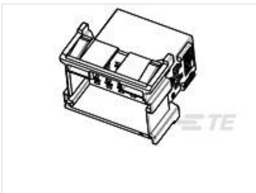
TE 产品编号1-967629-3 FLACHSTE-GEH2,8 18P
