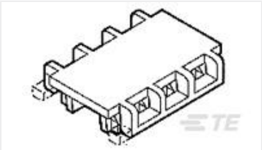
TE 产品编号643071-2 02P MTA156 FD-THRU COVER
