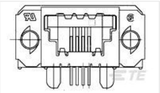
TE 产品编号5-1761185-3 8 SDL SE GRND RCPT ASSY
